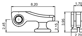
180° INSERT HINGE 03FR27223000
