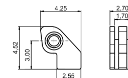
STEP HINGE 03FR27221000
