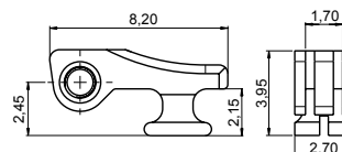
180° INSERT HINGE 03FR27223000
