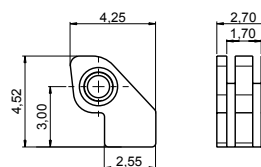
STEP HINGE 03FR27221000
