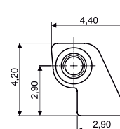
STEP HINGE 03FRC4163A1BY0
